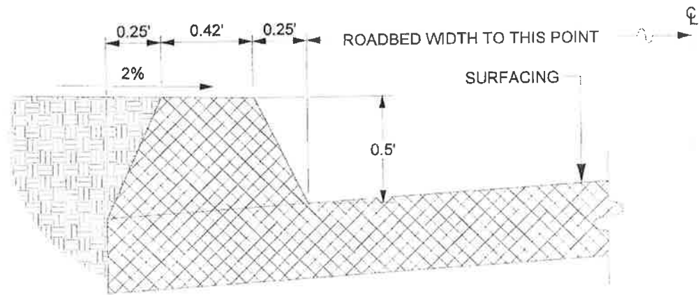
6" A.C. DIKE
