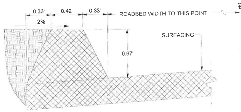
8" A.C. DIKE
