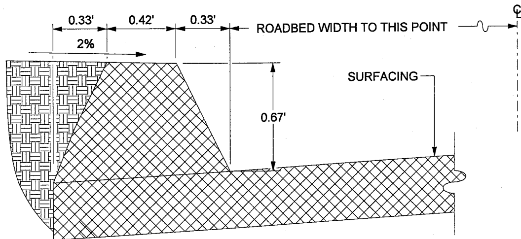
8" A.C. DIKE
