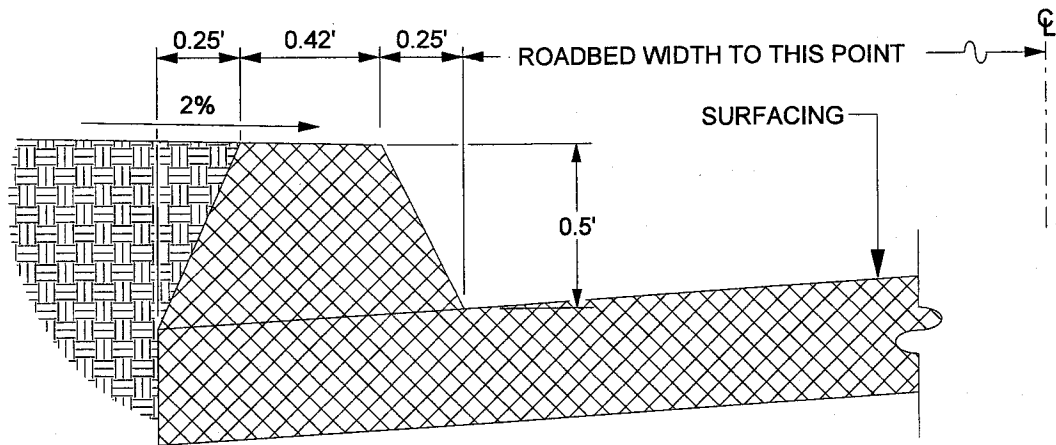
6" A.C. DIKE
