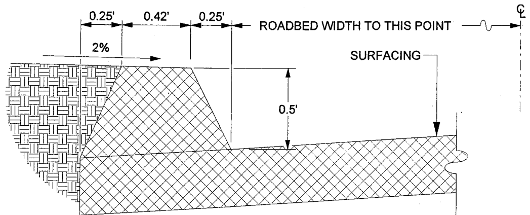
6" A.C. DIKE
