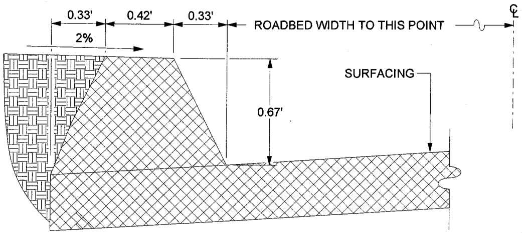
8" A.C. DIKE
