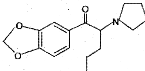
(MDPV)
