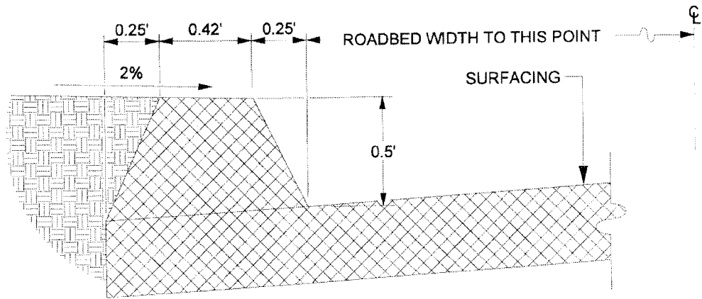
6" A.C. DIKE
