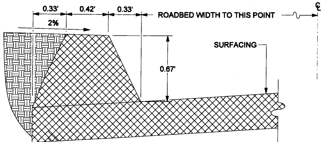
8" A.C. DIKE
