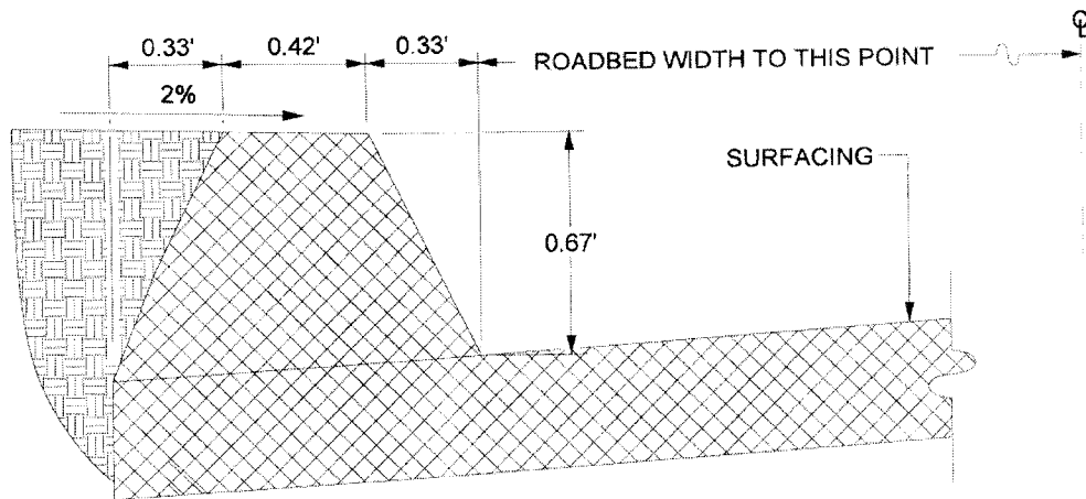
8" A.C. DIKE
