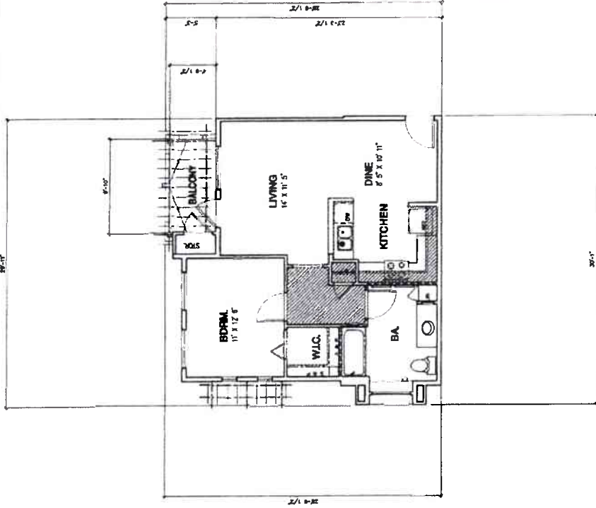
UNIT A2 1 BEDROOM - 1 BATH SCALE: 1/4" = 1'-0"
