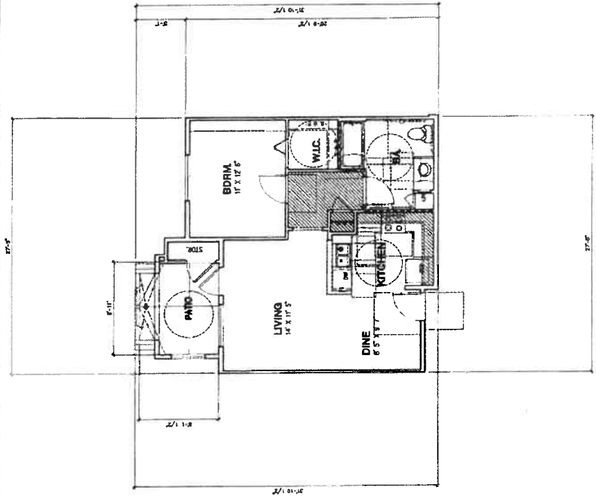
UNIT A11 1 BEDROOM - 1 BATH SCALE: 1/4" = 1'-0"
