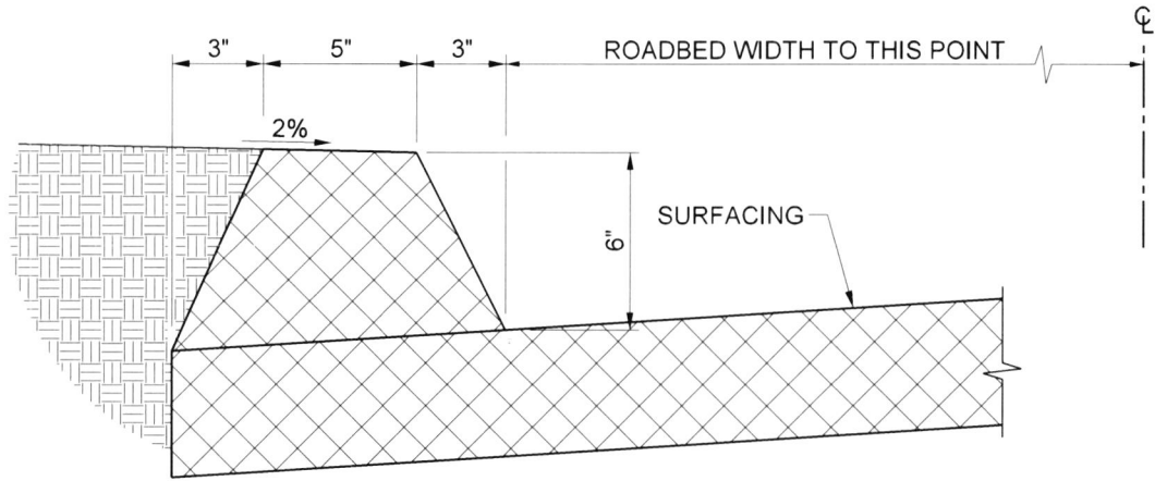
6" HMA DIKE
