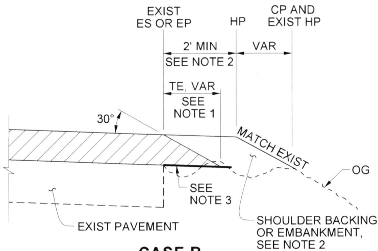
CASE B TAPERED EDGE
