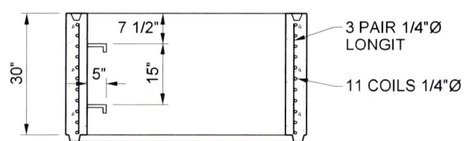
48" x 30" MANHOLE PIPE
