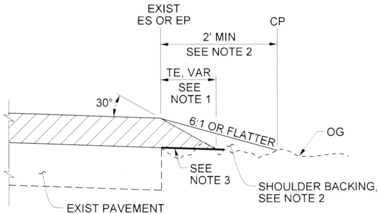
CASE A TAPERED EDGE
