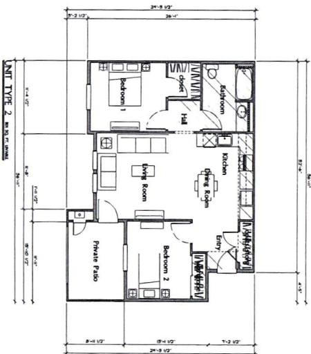
UNIT TYPE 2a
