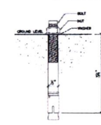
ANCHORING DETAIL SCALE: N.T.S.
