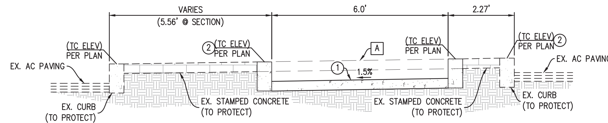
SECTION A-A
